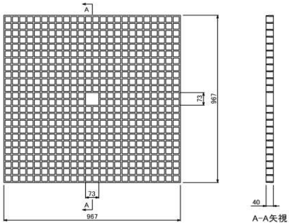
グリーンパネル 標準構造図
