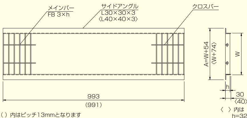
使用等辺山形鋼の寸法
