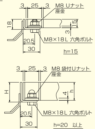
■ボルト固定詳細図
