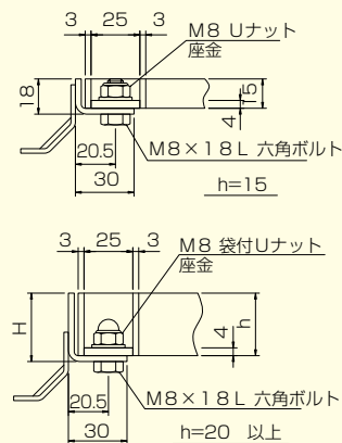
■ボルト固定詳細図
