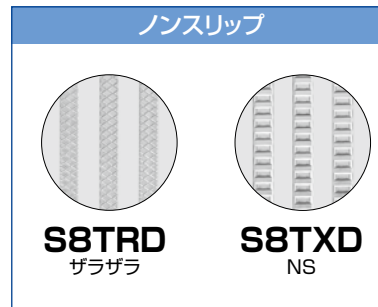
■ピッチ詳細図
