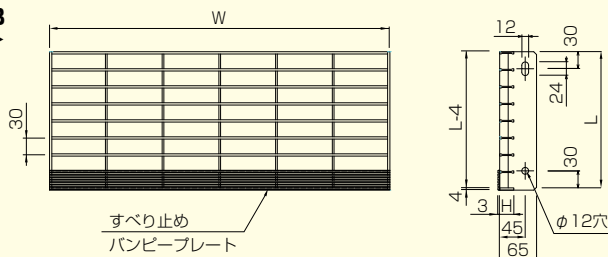
S4IF-SB <ボルト式>
