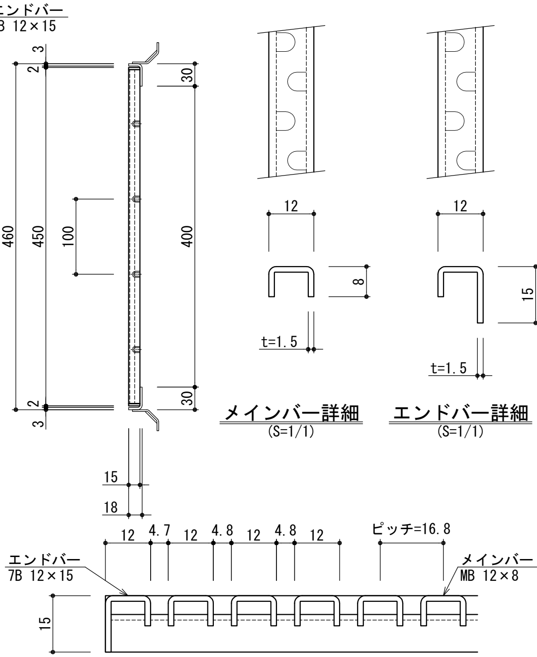
メインバー断面図 (S=1/1)
