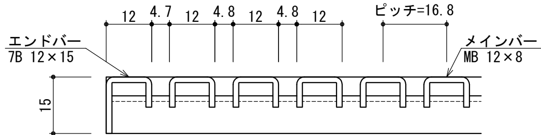
メインバー断面図 (S=1/1)
