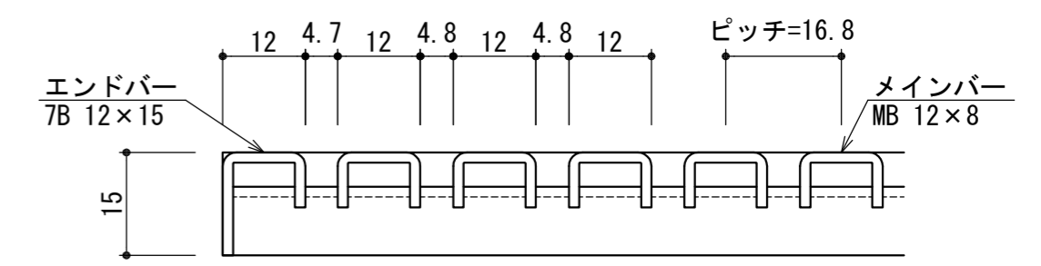
メインバー断面図 (S=1/1)
