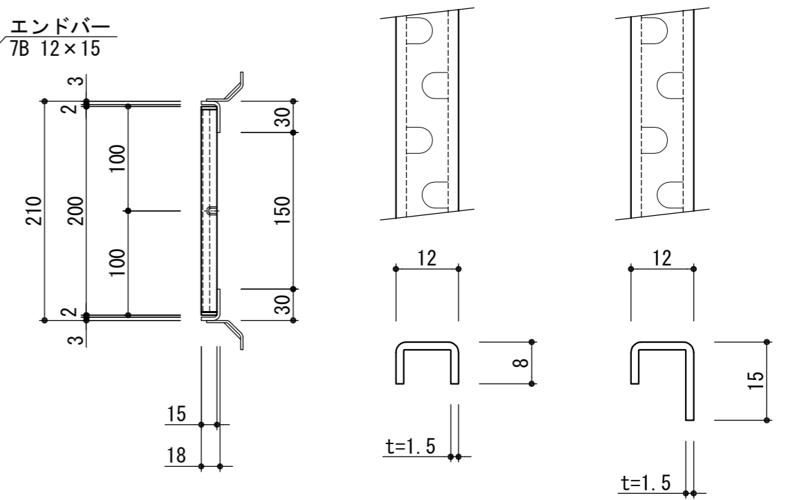
メインバー詳細 (S=1/1)
