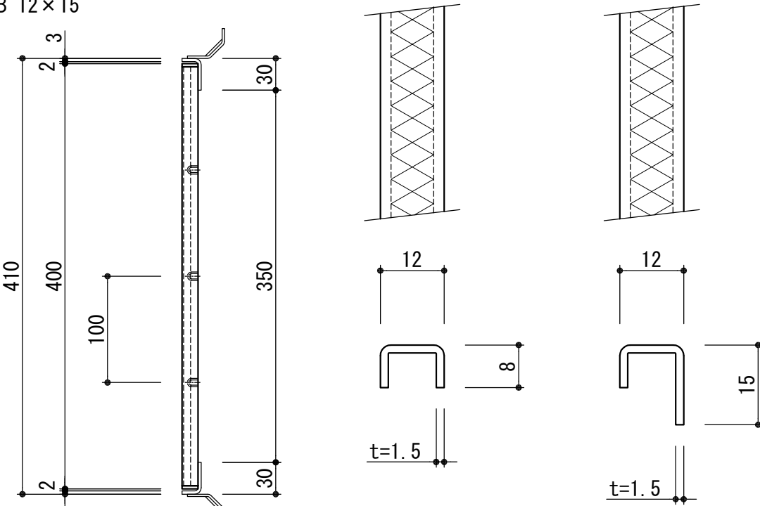
メインバー詳細 (S=1/1) エンドバー詳細 (S=1/1)
