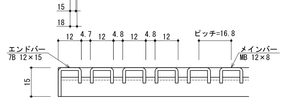
メインバー断面図 (S=1/1)
