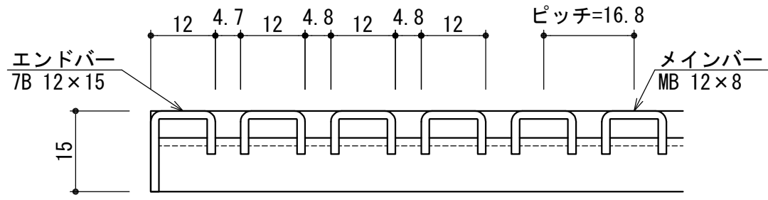
メインバー断面図 (S=1/1)
