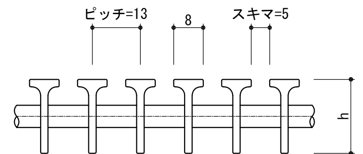
メインバー断面図 (S=1/1)
