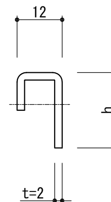
メインバー詳細 (S=1/1)
