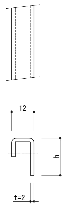
メインバー詳細 (S=1/1)
