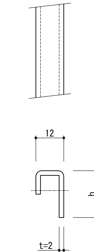
メインバー詳細 (S=1/1)
