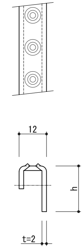
メインバー詳細 (S=1/1)
