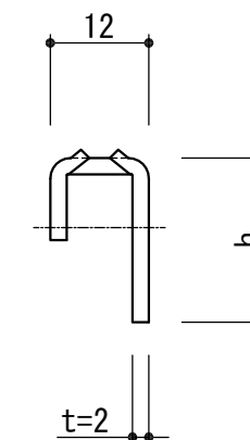
メインバー詳細 (S=1/1)
