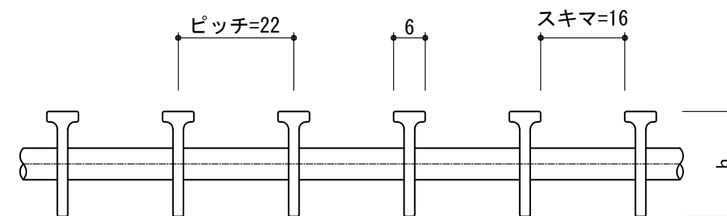
メインバー断面図 (S=1/1)
