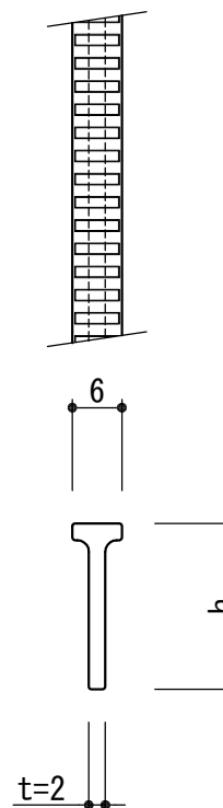
メインバー詳細 (S=1/1)
