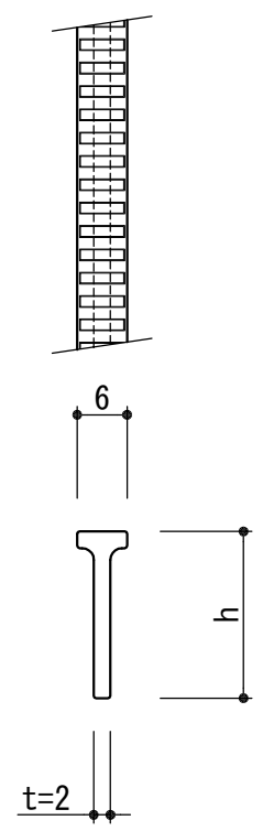
メインバー詳細 (S=1/1)
