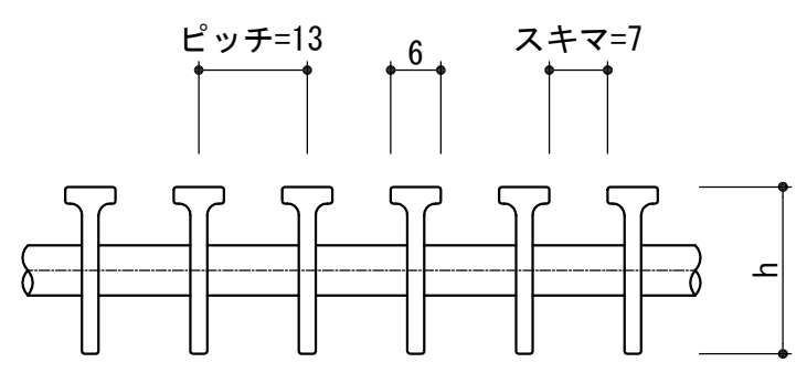
メインバー断面図 (S=1/1)
