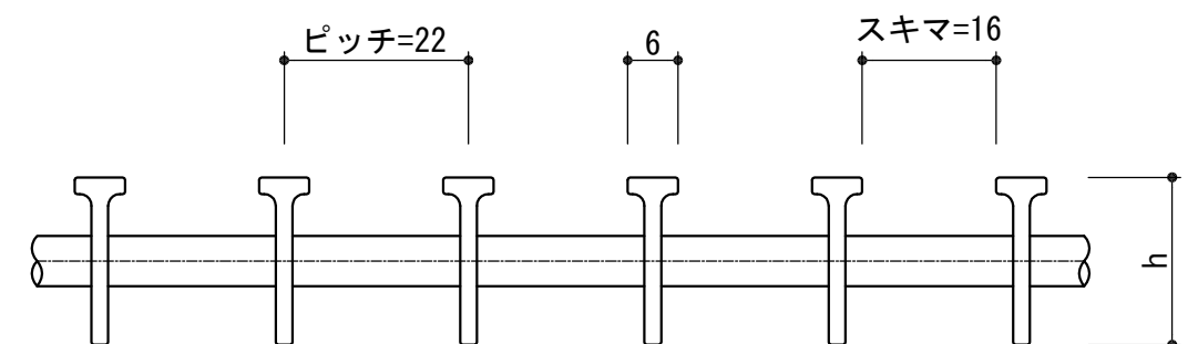
メインバー断面図 (S=1/1)
