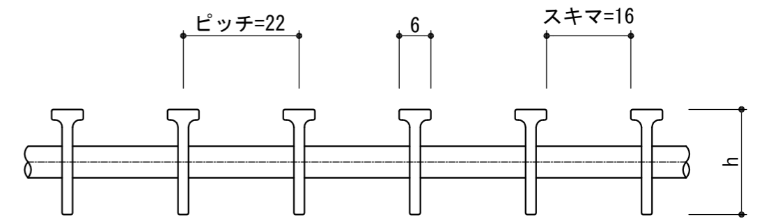
メインバー断面図 (S=1/1)
