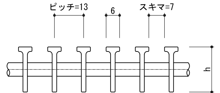
メインバー断面図 (S=1/1)
