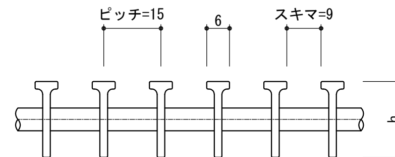
メインバー断面図 (S=1/1)
