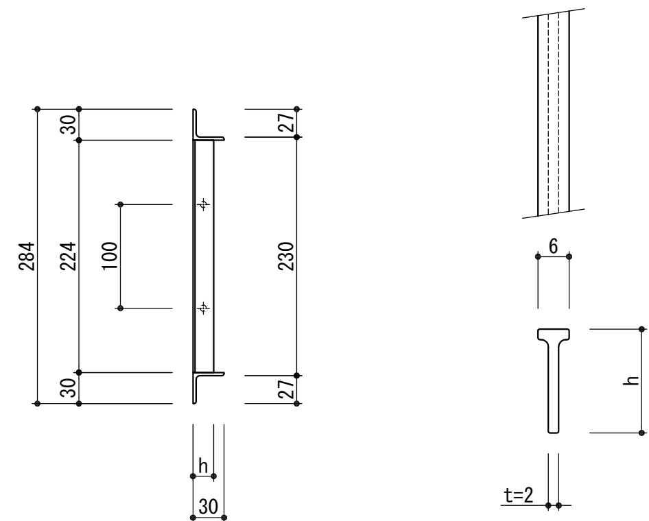
メインバー詳細 (S=1/1)
