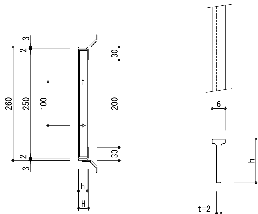
メインバー詳細 (S=1/1)
