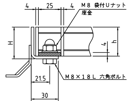
ボルト固定部詳細
