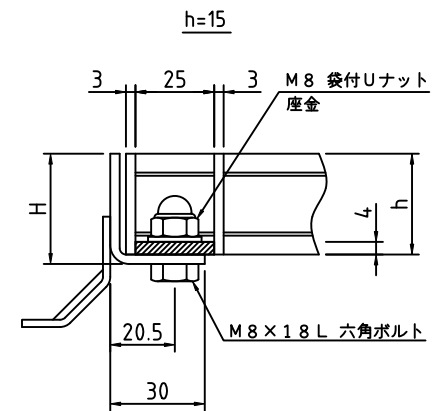
h=15 h=20 以上 ボルト固定部詳細
