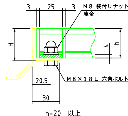
ボルト固定部詳細
