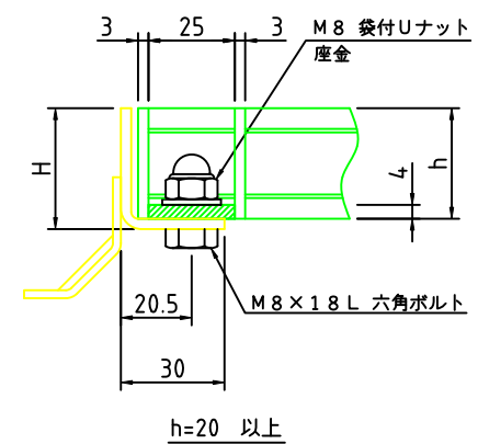
ボルト固定部詳細
