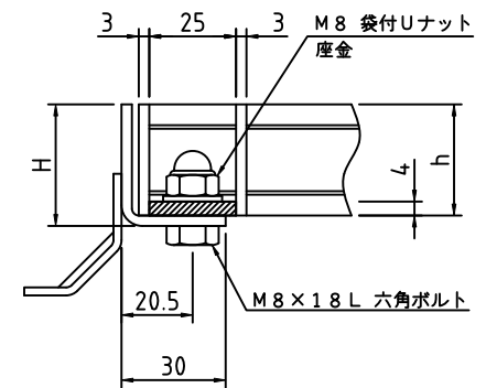
h=15 h=20 以上 ボルト固定部詳細
