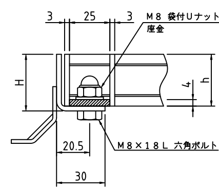
h=15 h=20 以上 ボルト固定部詳細
