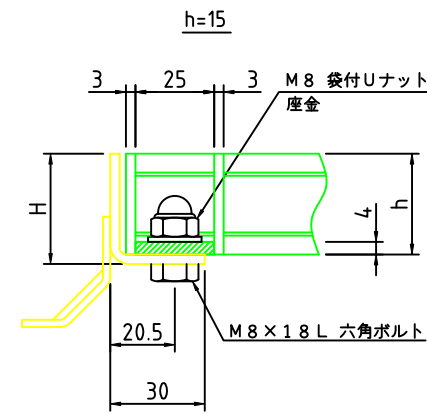
h=15 h=20 以上 ボルト固定部詳細
