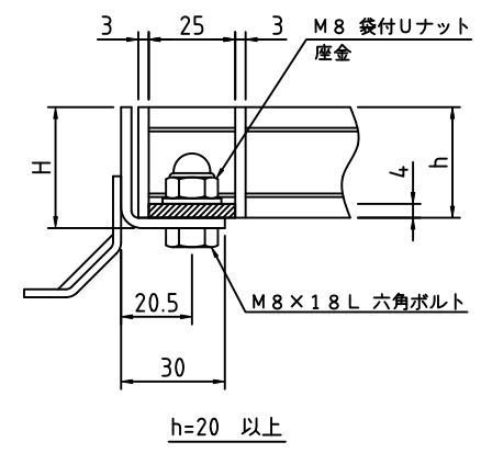
ボルト固定部詳細
