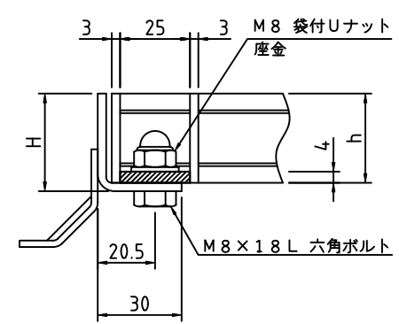
h=15 h=20 以上 ボルト固定部詳細
