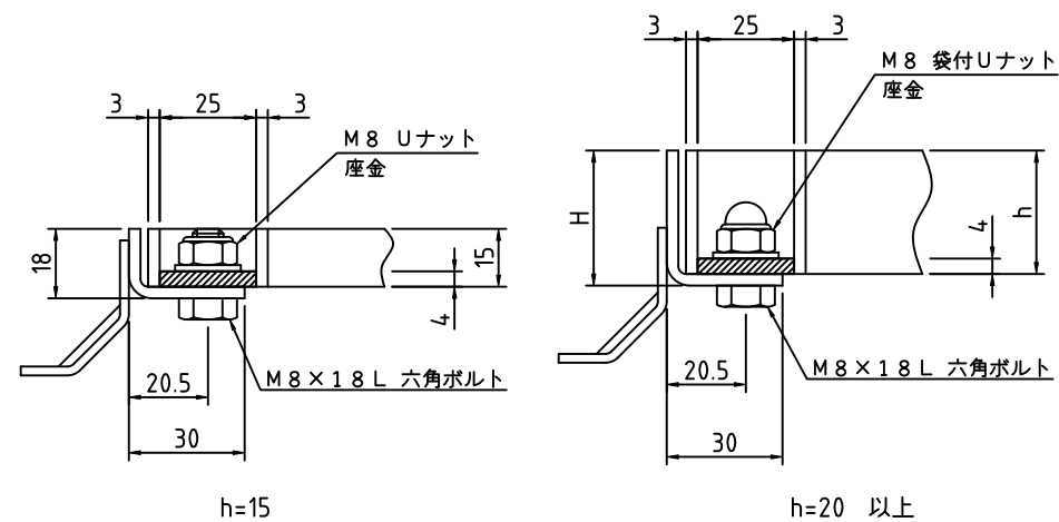
ボルト固定部詳細
