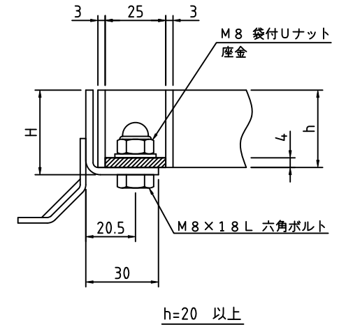
ボルト固定部詳細
