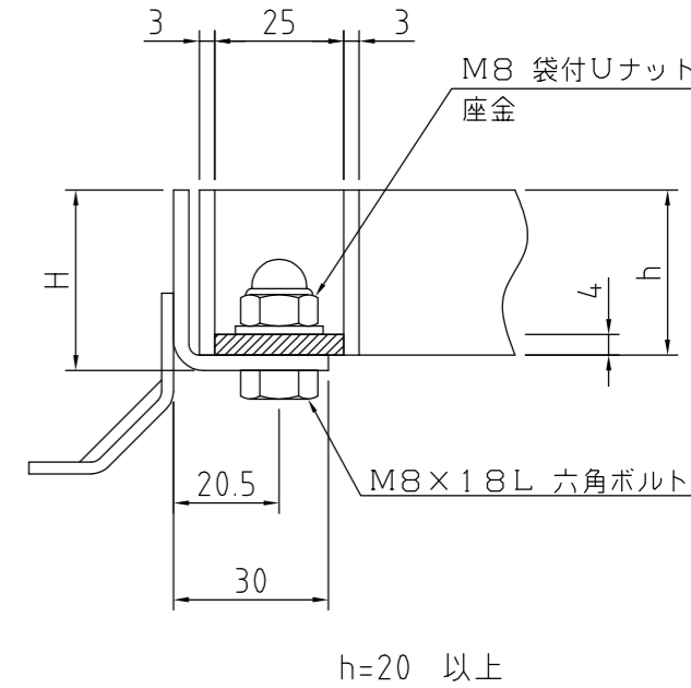
ボルト固定部詳細
