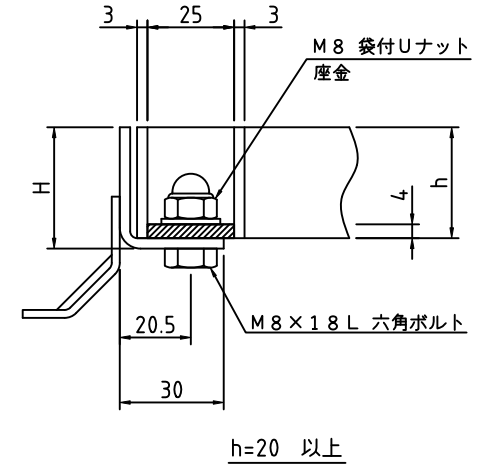
ボルト固定部詳細
