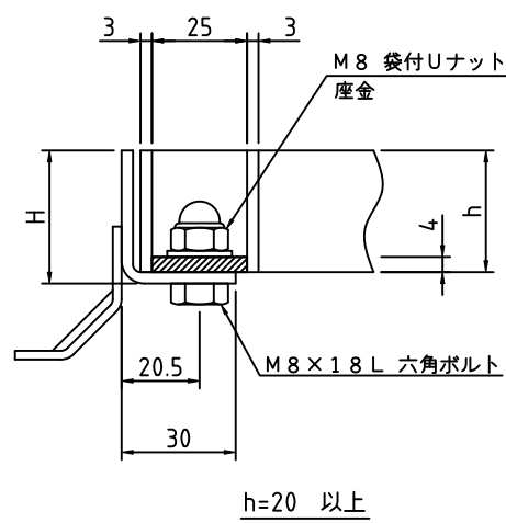
ボルト固定部詳細
