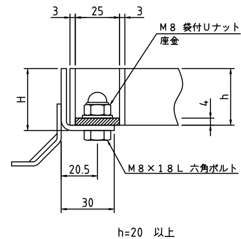
ボルト固定部詳細
