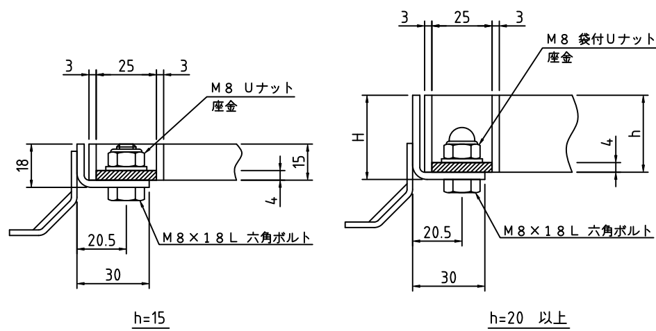
ボルト固定部詳細
