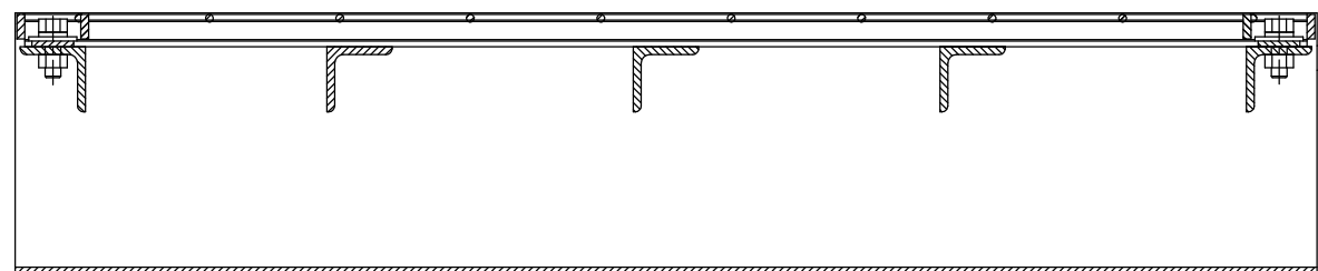
A-A断面図
