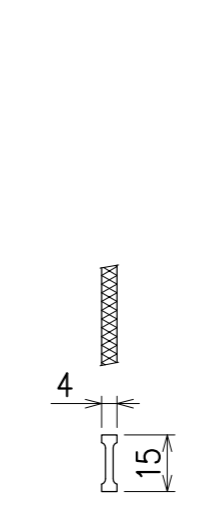
メインバー詳細 (ガラガラ)
