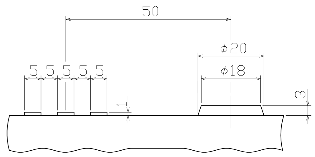
A-A すべり止め詳細図
