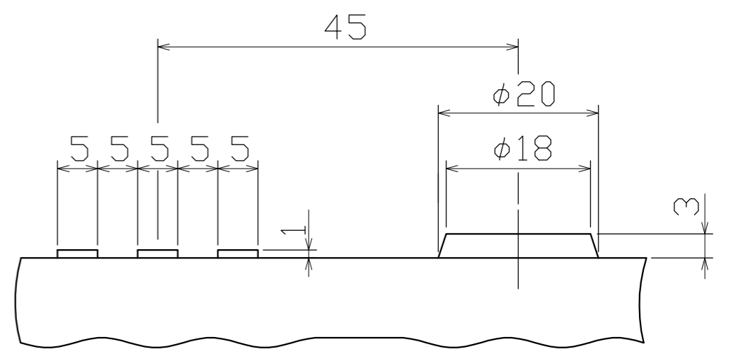
A-A すべり止め詳細図
