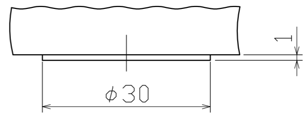
B部 裏面突起詳細図
