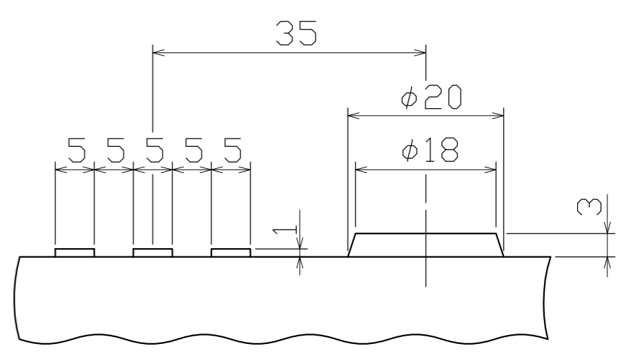
A-A すべり止め詳細図
