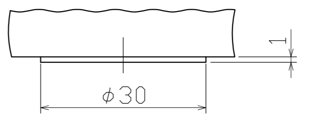
B部 裏面突起詳細図
