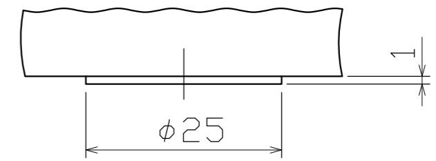
B部 裏面突起詳細図
