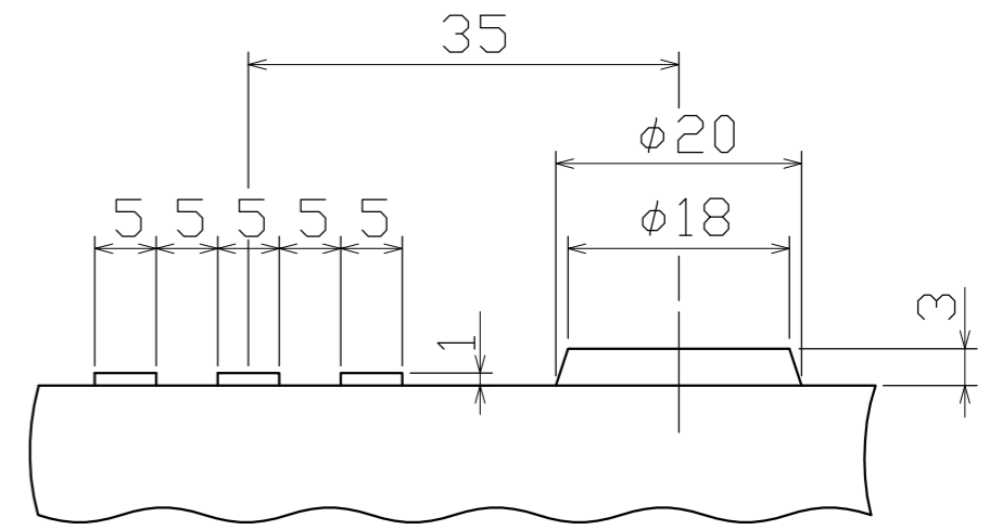
A-A すべり止め詳細図
