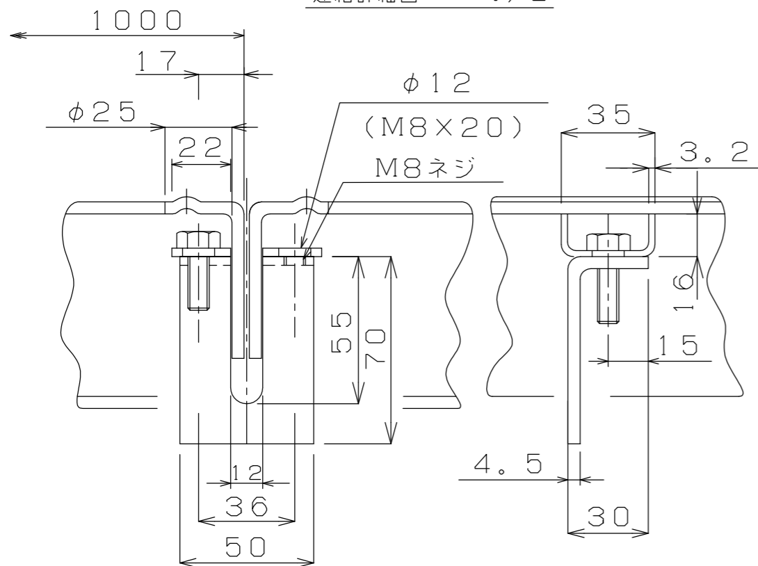
連結詳細図 S=1/2
