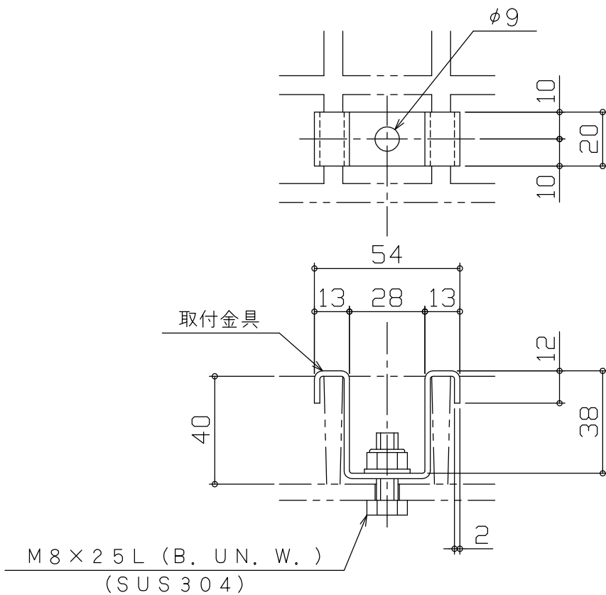
取付金具詳細 S = 1 / 2 PF - 2 型
