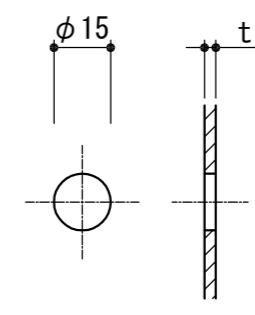
水抜孔詳細 (Eタイプ) (S=1/2)
