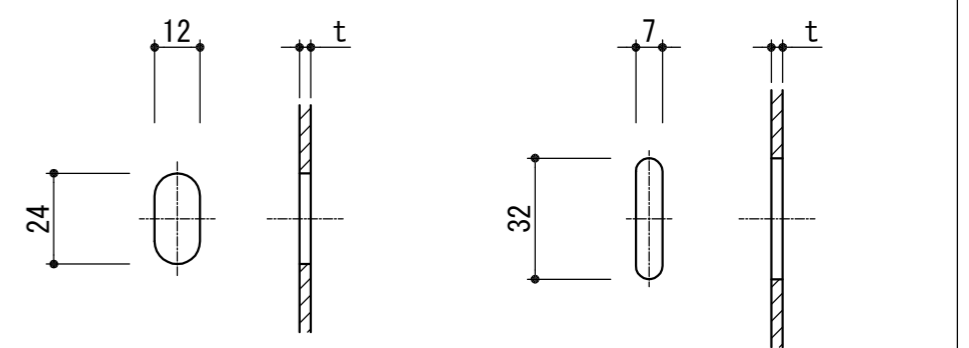
水抜孔詳細 (Aタイプ) (S=1/2)
